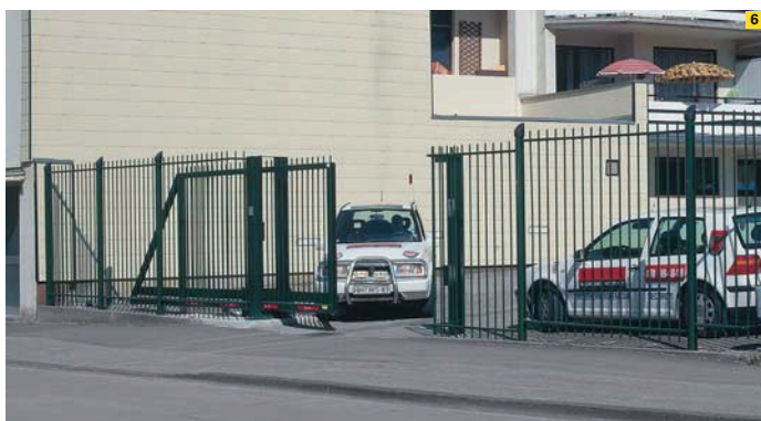
6. adronit®-Stabzaun SIGURA in Kombination mit dem freitragenden adronit®-Schiebetor ATLAS SL und passender SIGURA-Füllung
